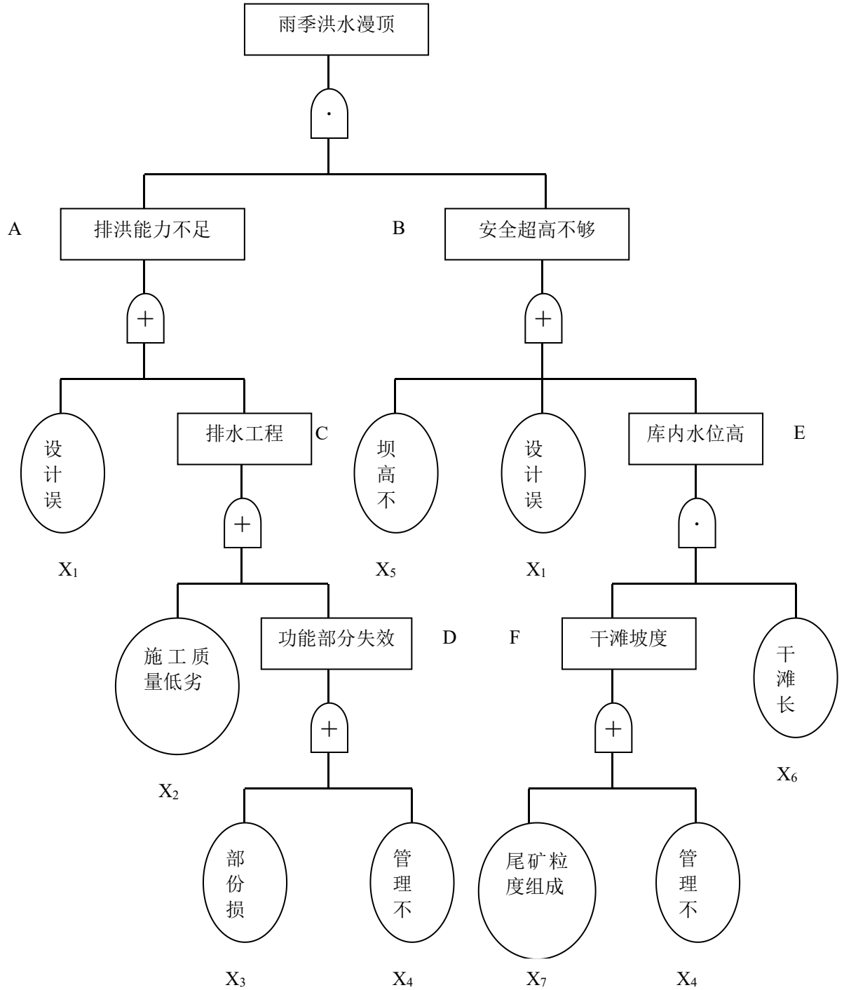
图 5-2 事故树图
