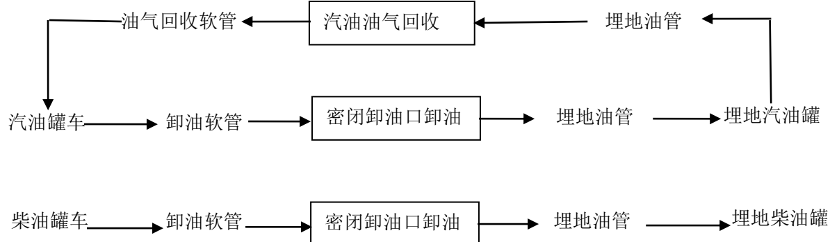
图 2.6-1 汽车卸油工艺流程图
